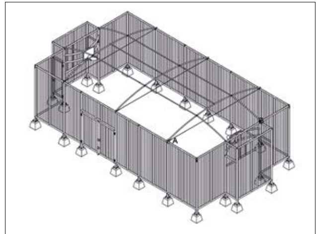
Dachnetz mit gebogener Dachkonstruktion
