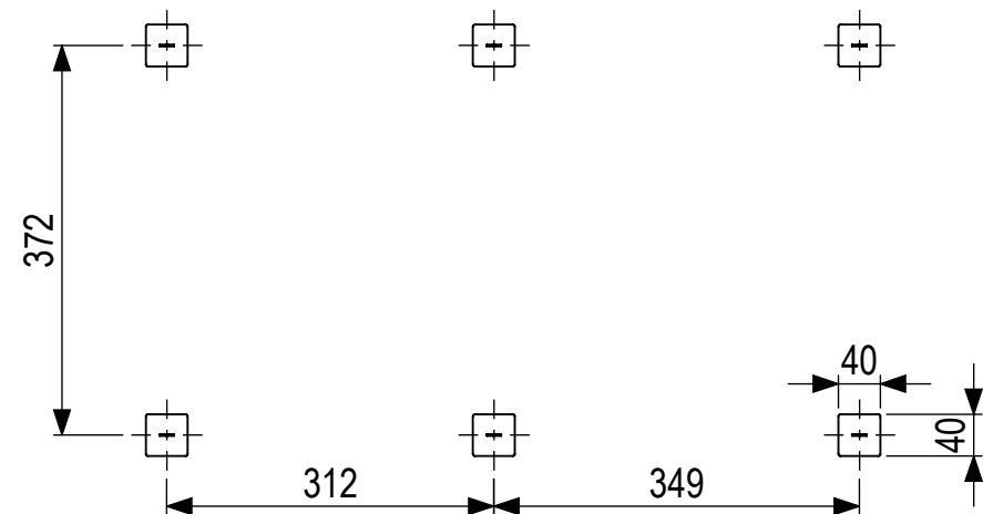
Voetplan SCALE 1:80
