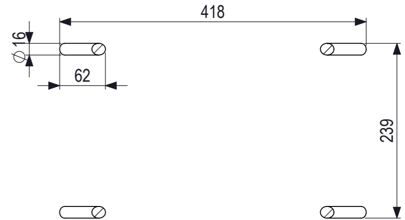
Voetenplan
