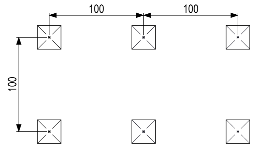
Fundatieplan
